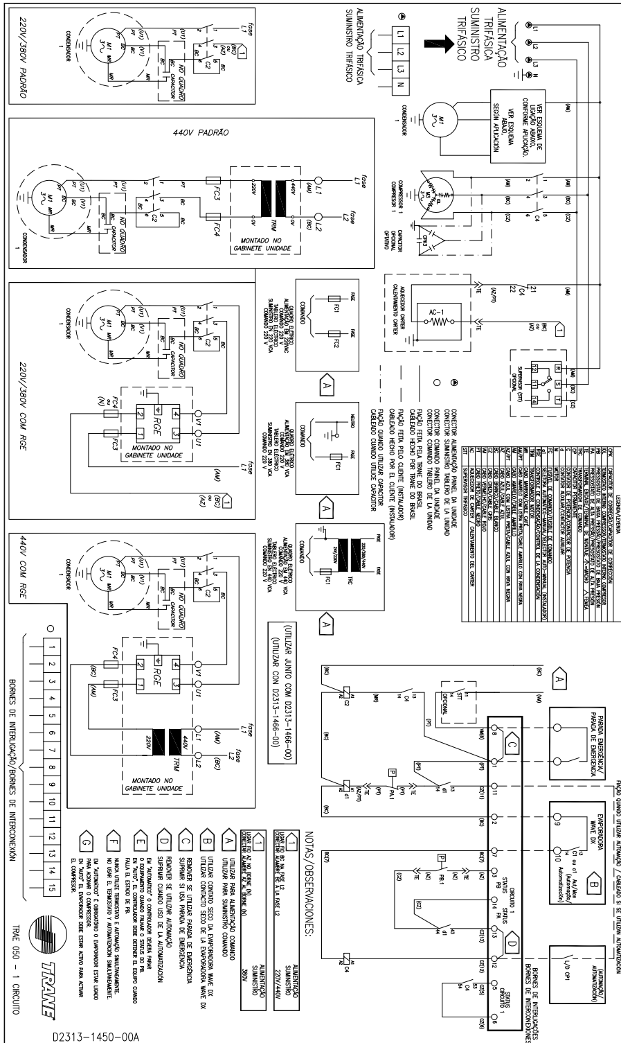
Fig. VII-01 - Wiring Diagram - TRAE050
