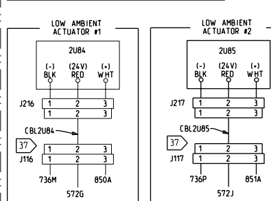
INSET "3AB"- OPTIONAL LOW AMBIENT DAMPER ACTUATOR
