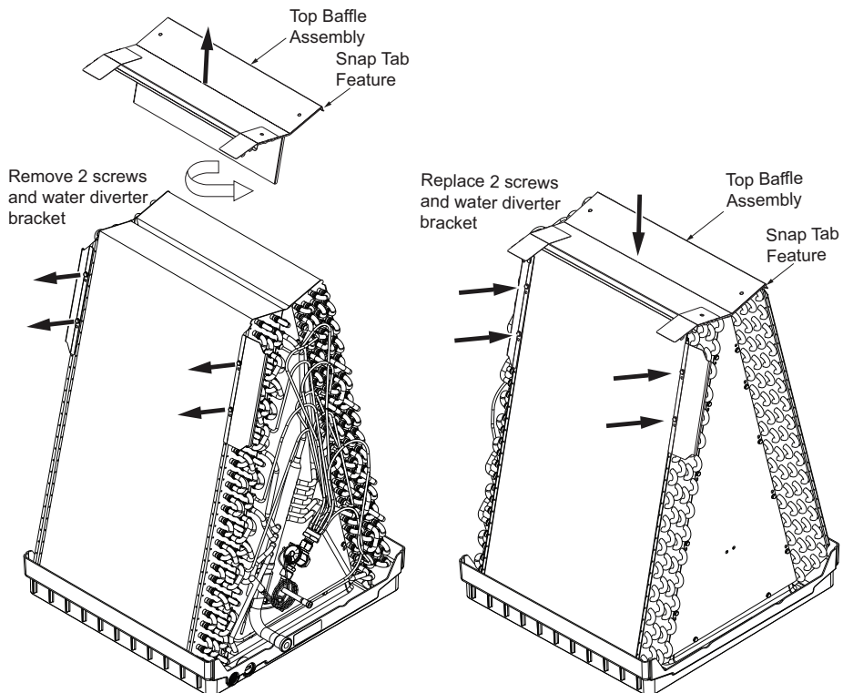
Figure 21. A4AH5E49A1C30AA, A4AH5E61A1C30AA, A4AH5V48A1C30AA, A4AH5V60A1C30AA
