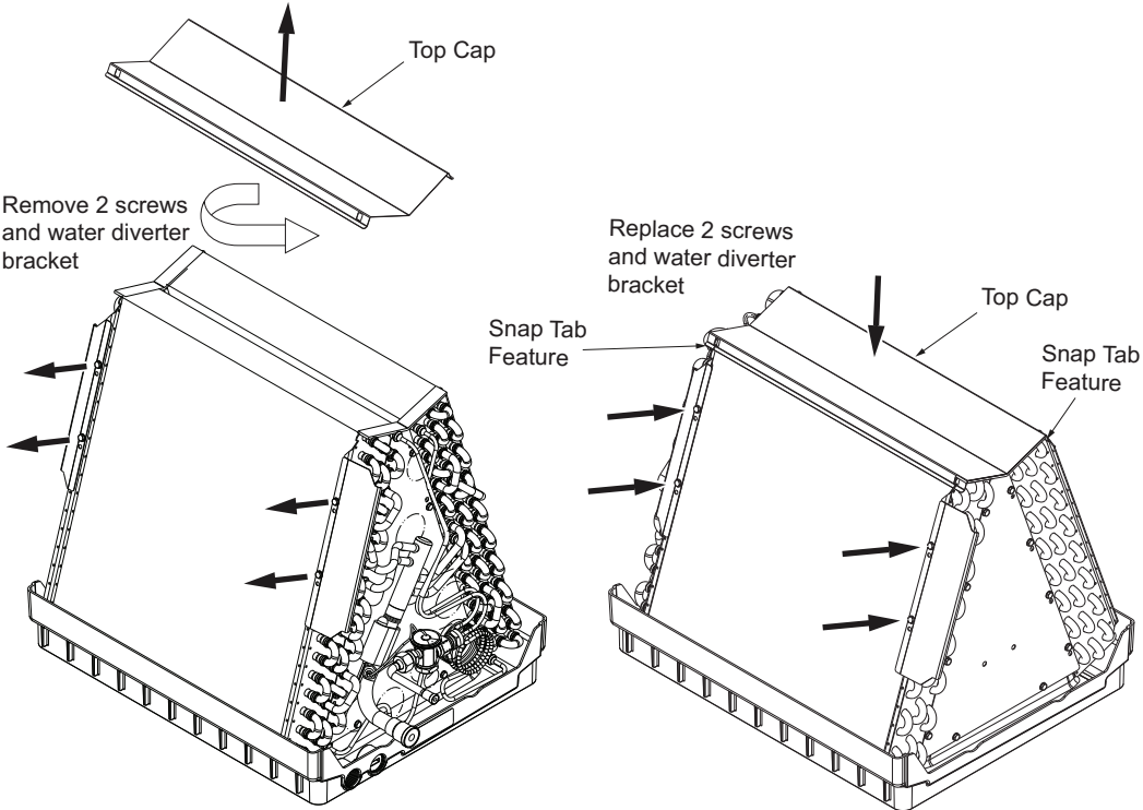
Figure 19. A4AH5E31A1B30AA, A4AH5V24A1B30AA, A4AH5V30A1B30AA
