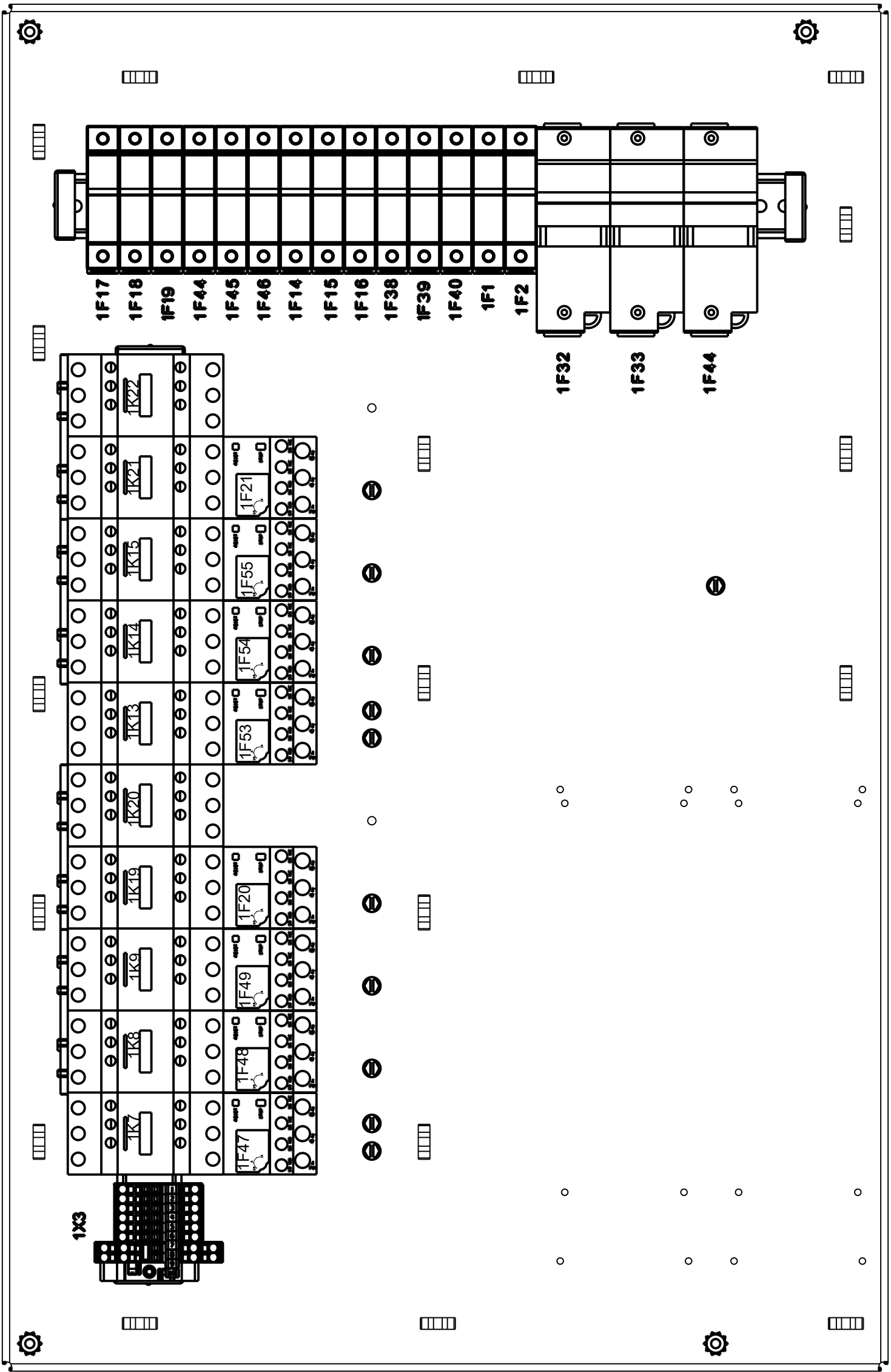
DETAIL C WO VFD 2SP, 3 FANS/CKT
