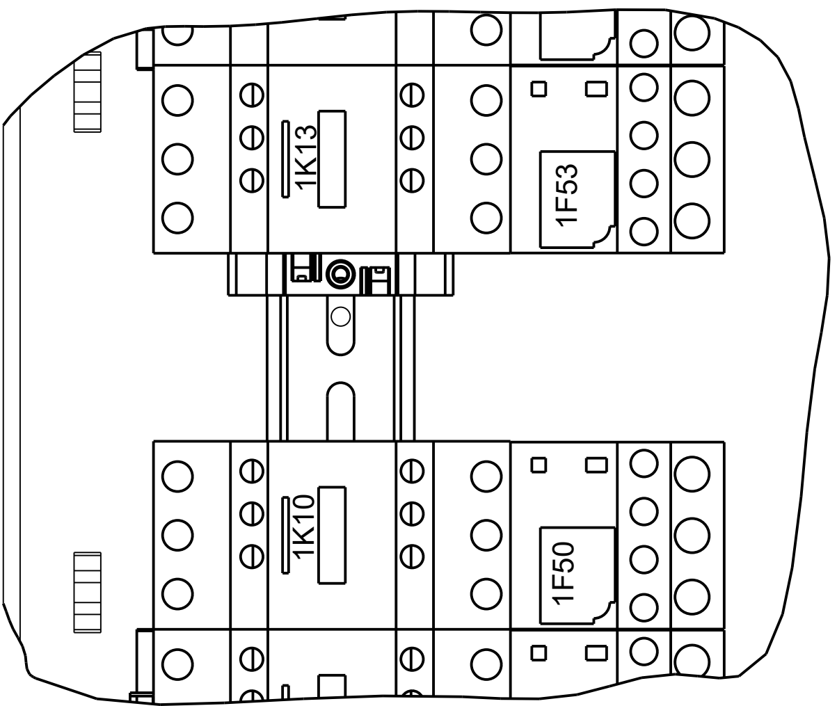
DETAIL D WO VFD 1 SP, 4 FANS/CKT
