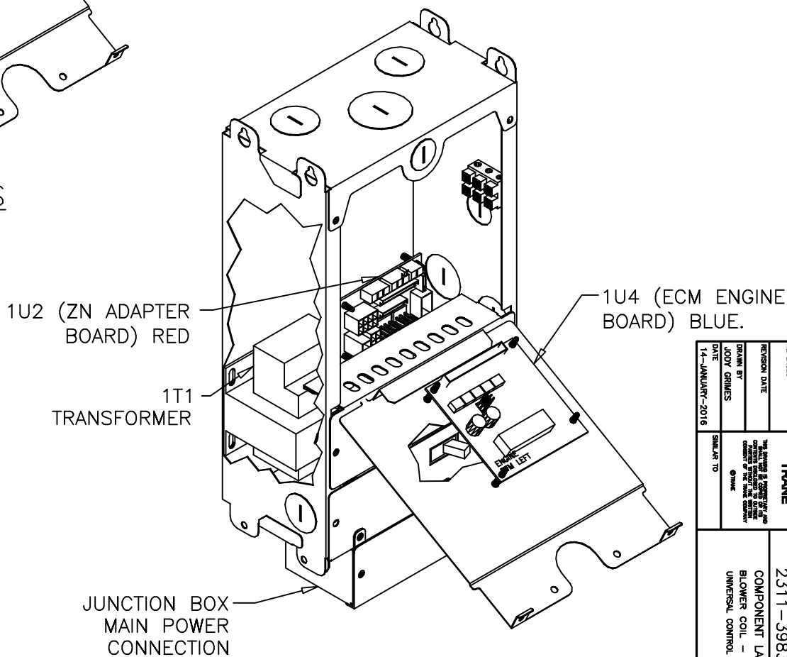
FAN SPEED SWITCH CONTROLS
