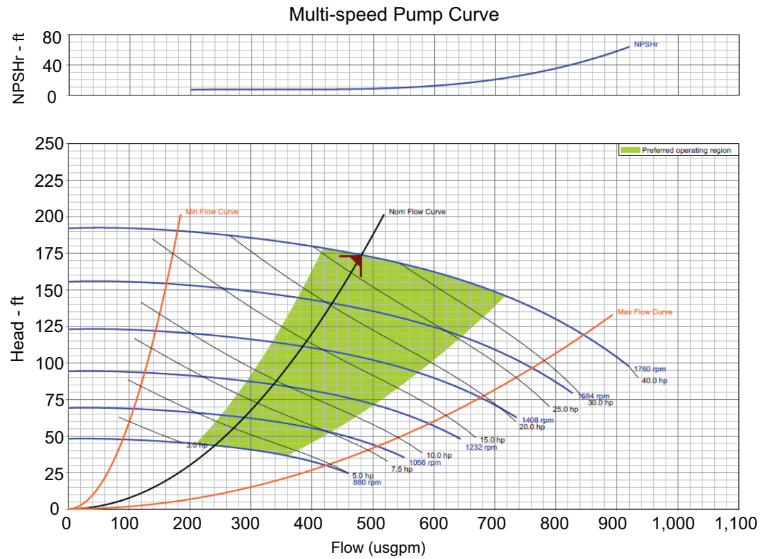
Figure 35. 200 ton ACSA (F0 to F1)/200 ton AXCA (F1) — multi speed
