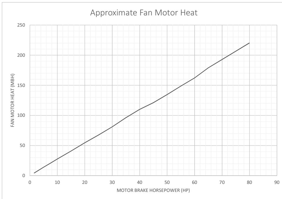
Figure 6. Fan motor
