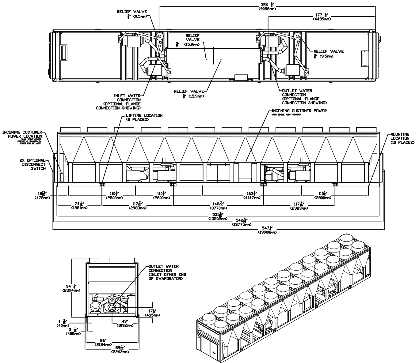
Figure 10. RTAF unit dimensions — 410 ton
