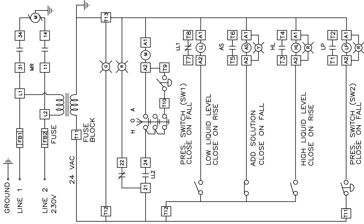
WIRING SCHEMATIC
