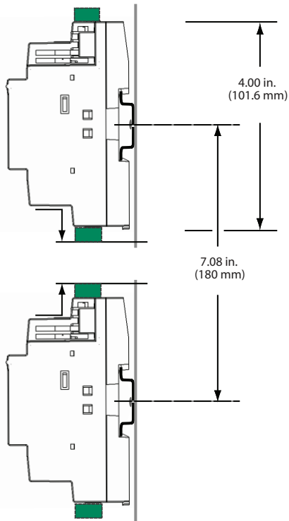
Figure 3. DIN Rail
