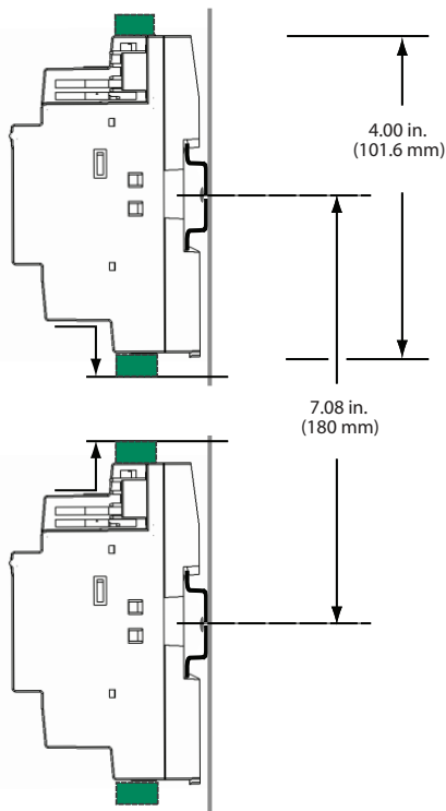
Figure 3. DIN Rail
